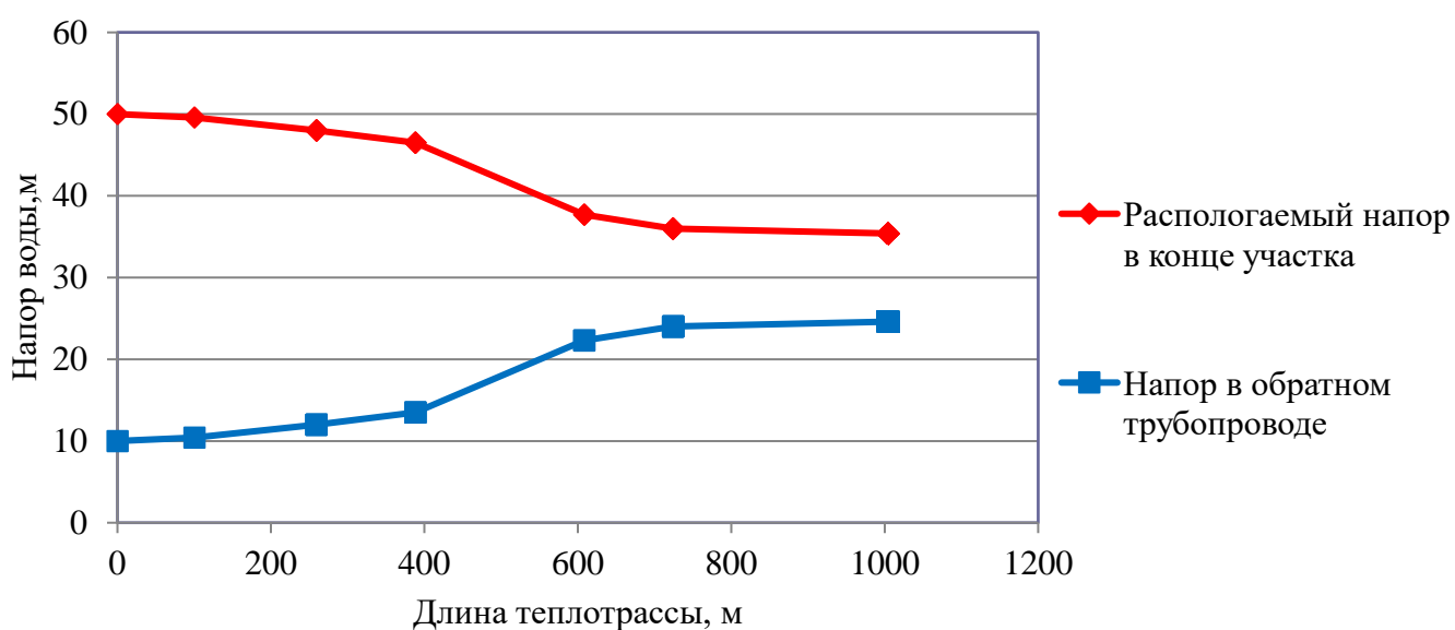
Рисунок 2.21 – Пьезометрический график тепловой сети Котельная п. Нагорный до ул. Советская 14
