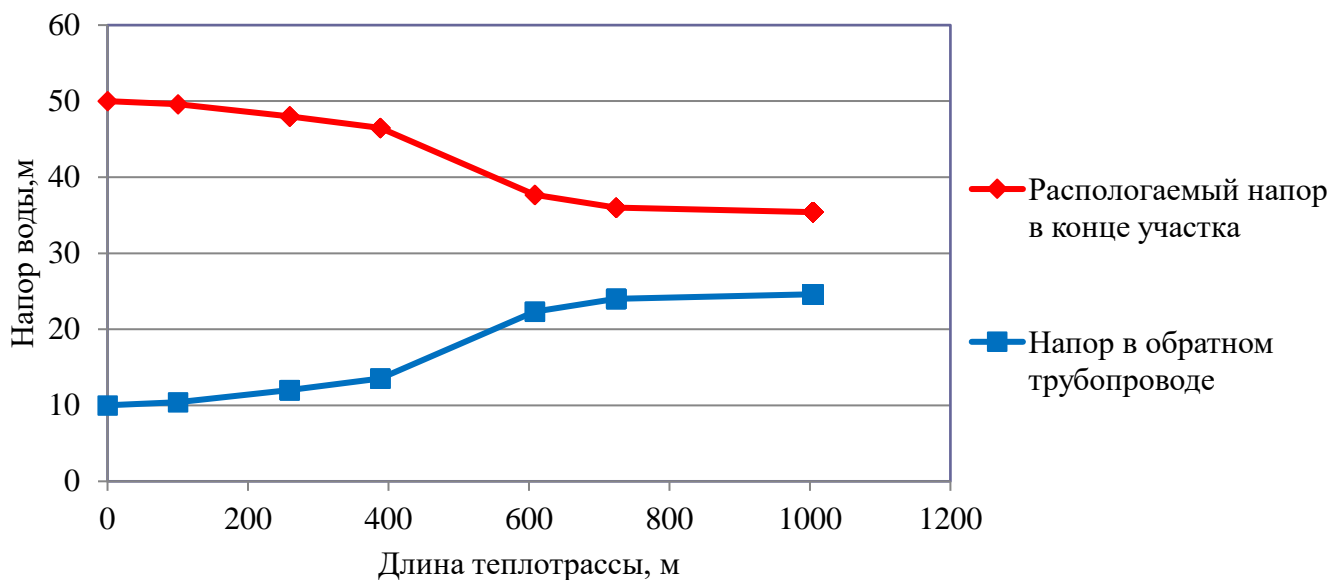
Рисунок 2.11 – Пьезометрический график тепловой сети Котельная п. Нагорный до ул. Советская, 14
