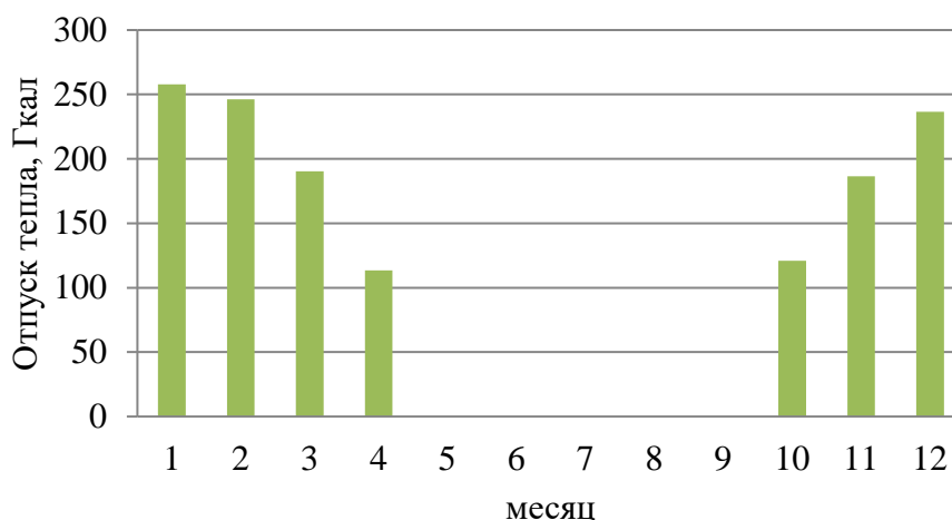
Рисунок 1.8 Оптимальный температурный график отпуса тепловой энергии для Котельная п. Нагорный с температурным режимом 90-70 °С
