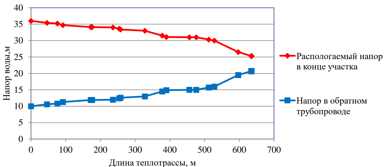
Рисунок 2.18 – Пьезометрический график тепловой сети Котельной №2 с. Кичигино до домов по ул. Крыдова
