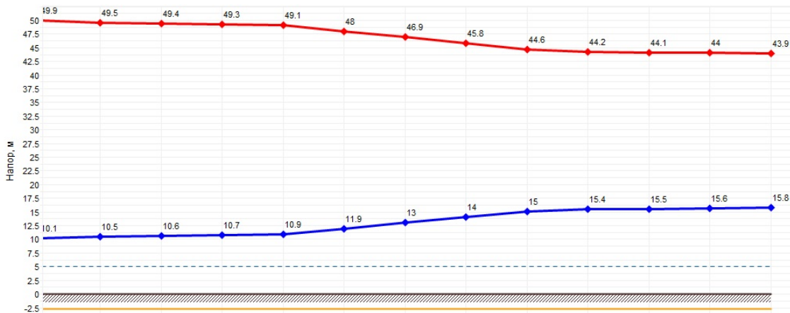
Рисунок 2.42 Пьезометрический график от Котельной п. Нагорный до самого удаленного потребителя в аварийной ситуации здания детского сада
