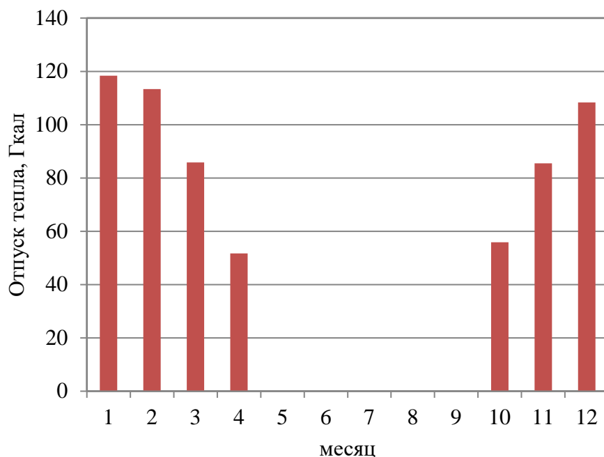
Рисунок 1.5 – Оптимальный температурный график отпуски тепловой энергии для Котельной №1 с. Кичигино с температурным режимом 85-64 °С
