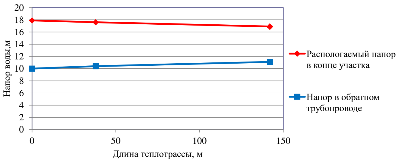
Рисунок 2.7 – Пьезометрический график тепловой сети Котельной №1 с. Кичигино
