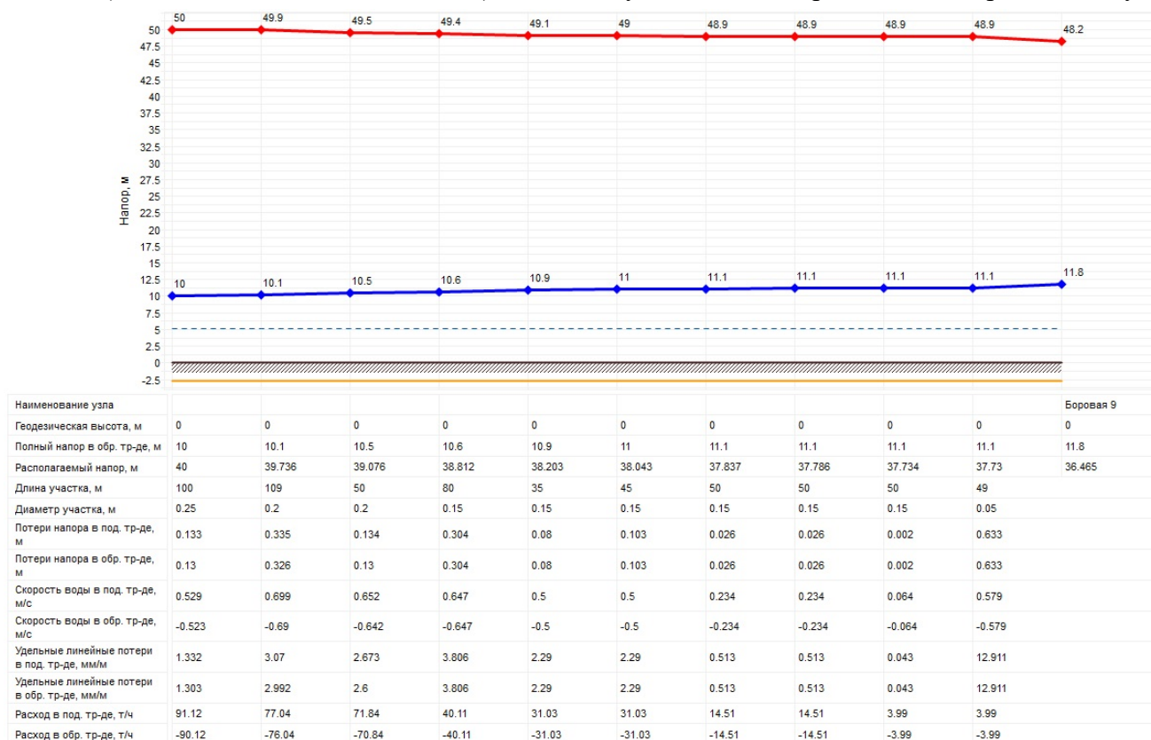
Рисунок 2.41 – Пьезометрический график от Котельной п. Нагорный до самого удаленного потребителя в аварийной ситуации по ул. Боровая
